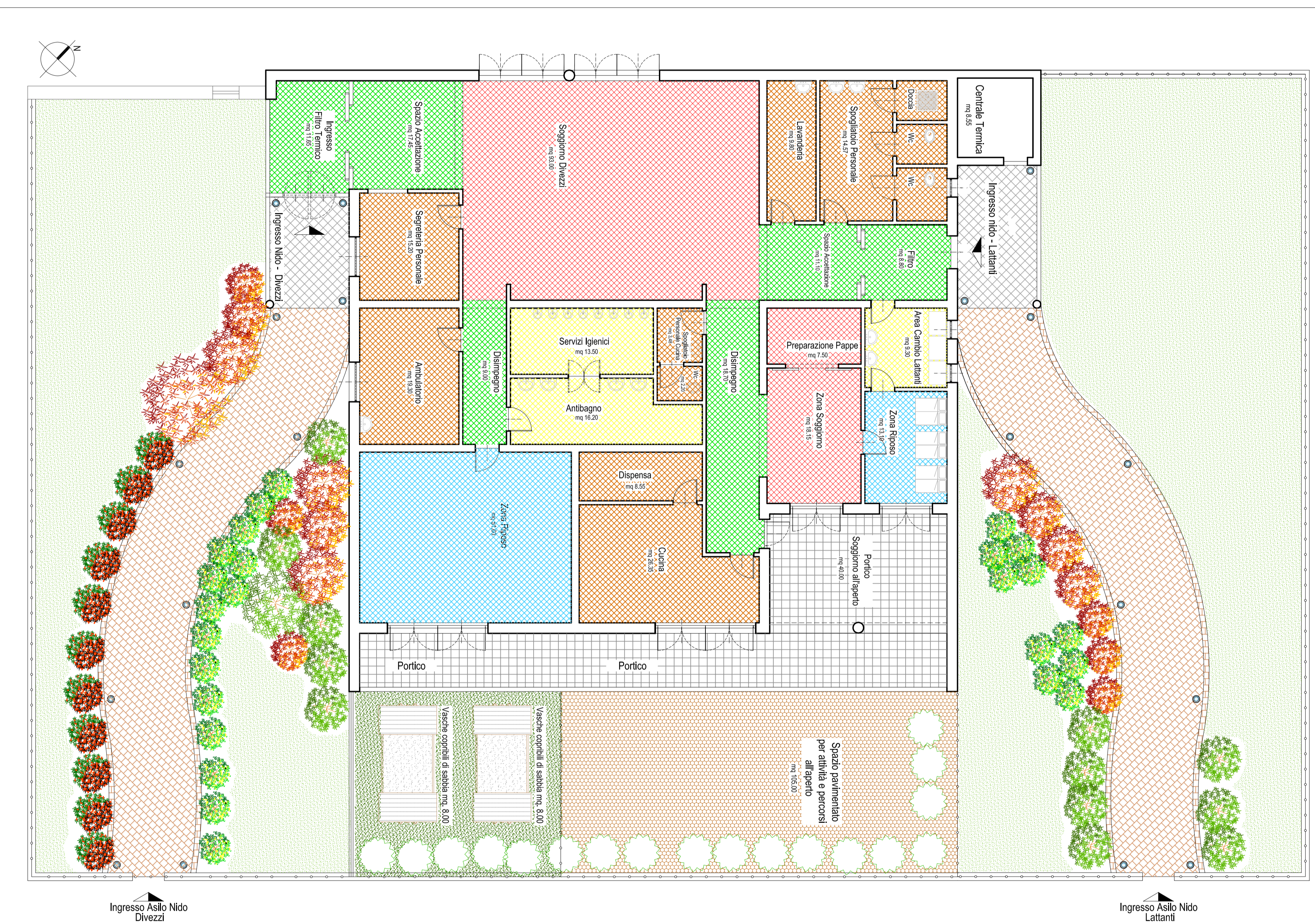
PANITA CON INDIVIDUAZIONE SPAZI A STANDARDS - scala 1:100
